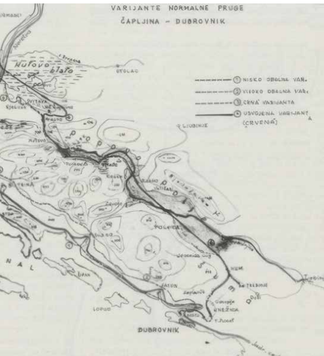
Varijante trase pruge Čapljina – Dubrovnik, Izvor: Časopis 'Građevinar', Zagreb, 6/1973, Oto Derner, dipl. ing. Sarajevo
